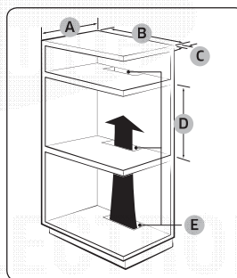
Отсек встроенной мебели (мм)
