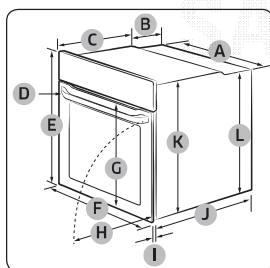
Духовой шкаф (мм)
