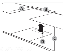
Шкаф под раковиной (мм)
