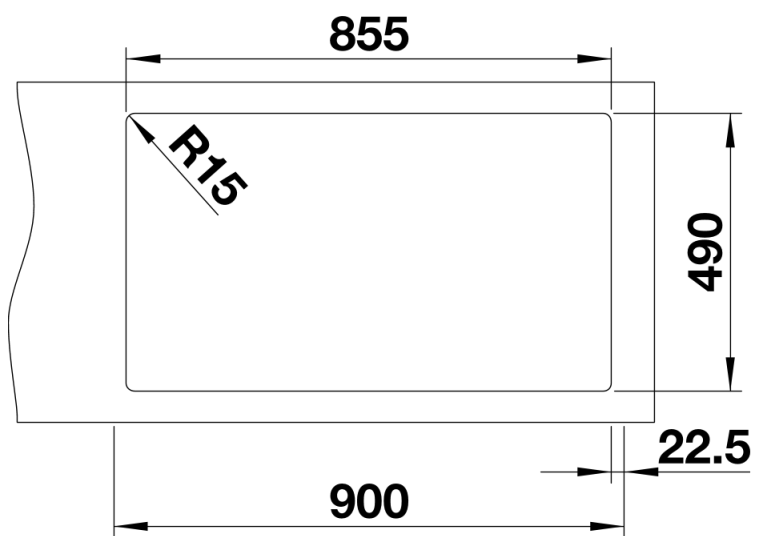
Вырез
