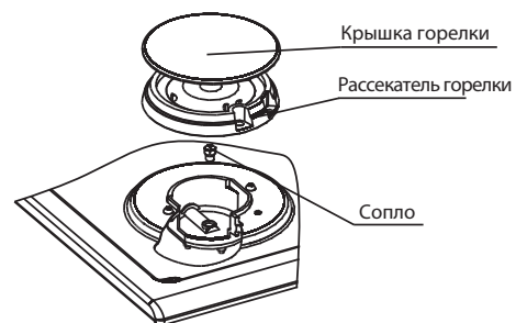
Замена сопла горелок стола
